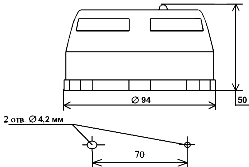
Рисунок 1 - Габаритные и установочные размеры извещателя
