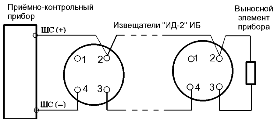
Рисунок 2 - Типовая схема включения извещателей
