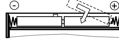
Установка второй пары элементов питания
