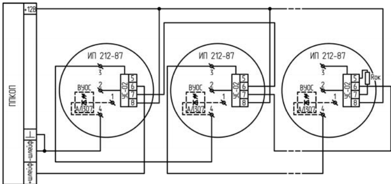
Схема подключения ВУОС
