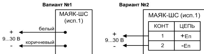
Рис.1 Схема подключения.
