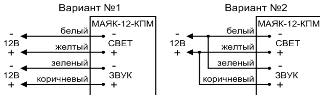
Рис.1 Схема подключения.
