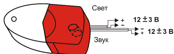
Рис.2 Схема подключения ПКИ-СП12.
